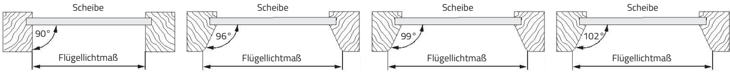
Fenster-Aufmaß (Spalte 5)
